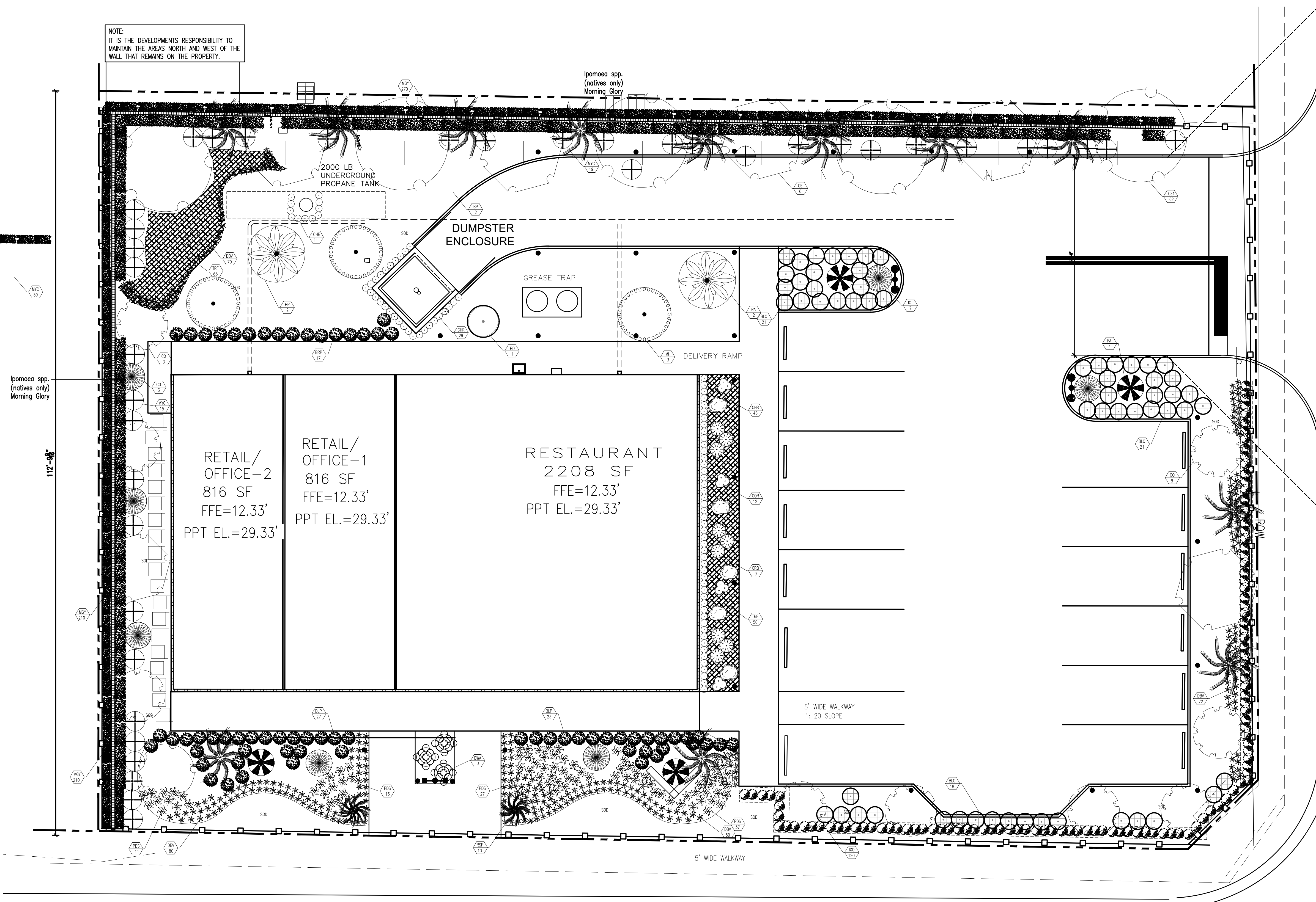
LANDSCAPING PLAN SCALE: 1/8" = 1'-0"
